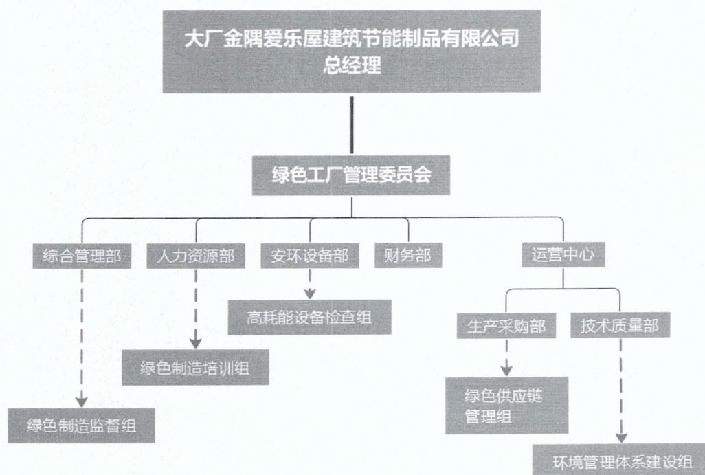
图 1-1 组织结构图
